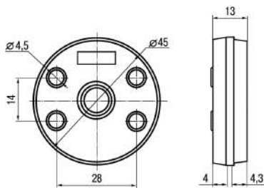
Рисунок 6.1 – Габаритный чертеж прибора
